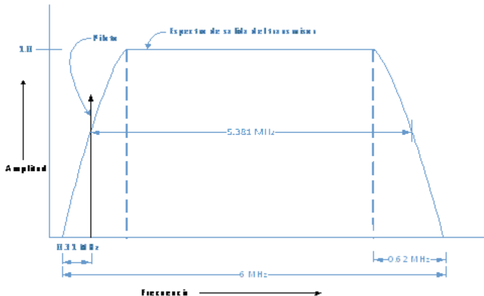
Figura 3. Características del Canal de Transmisión
